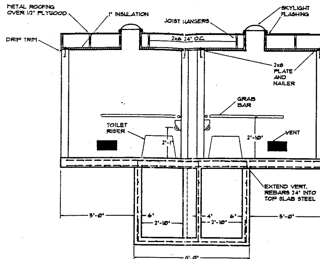
B 2 SECTION B SCALE: 1/4" = 1 FOOT
