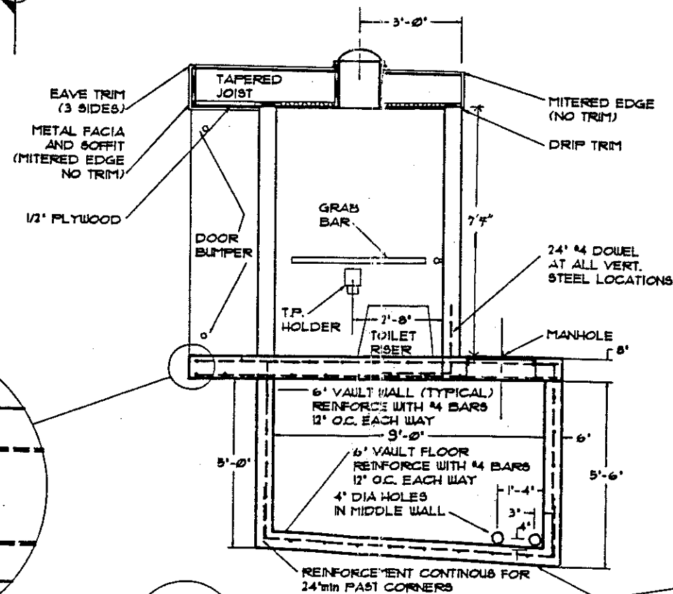
C 2 SECTION C SCALE: 1/8" = 1 FOOT
