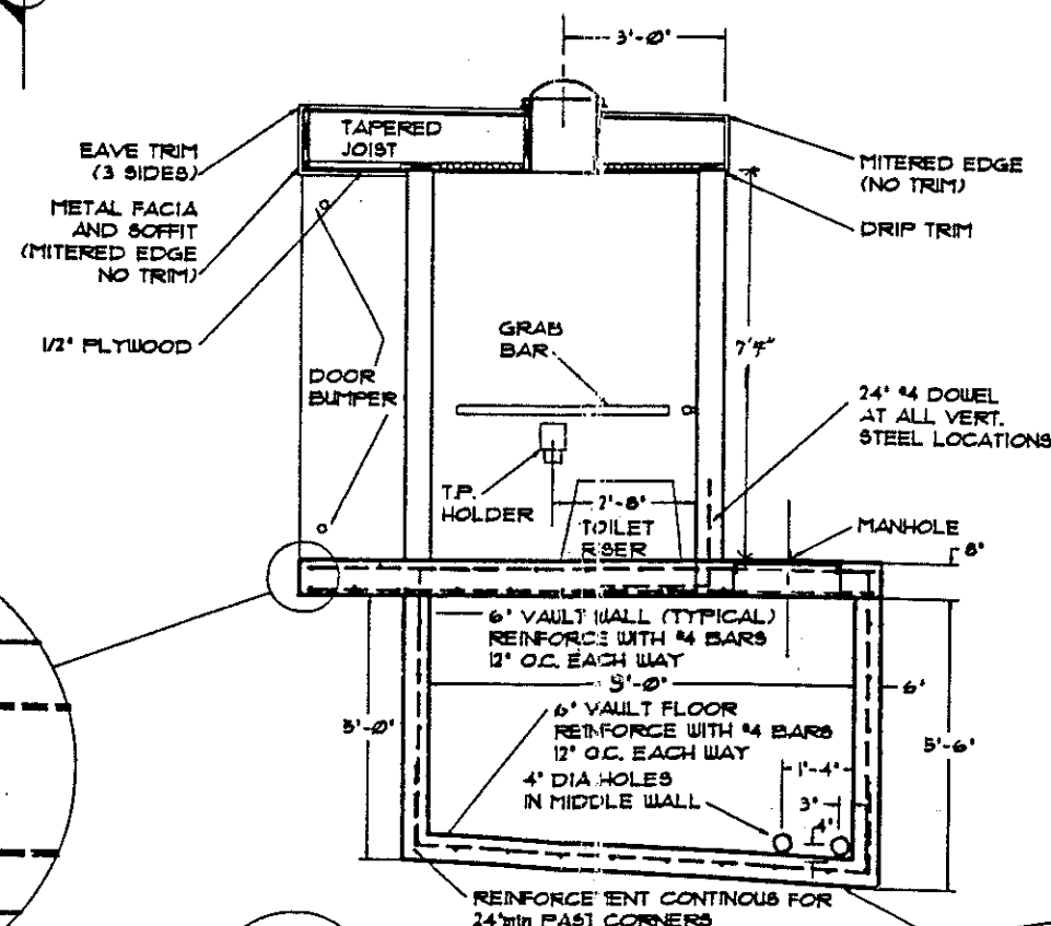
C 2 SECTION C SCALE: 1/4" = 1 FOOT
